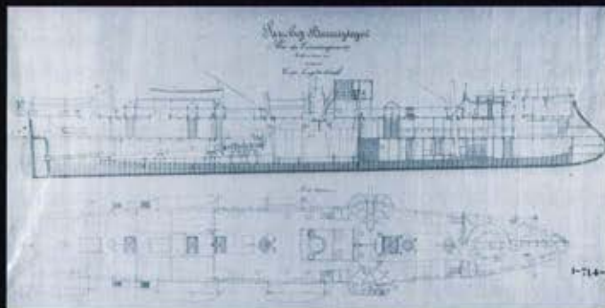
Plano del «Sánchez Barcaiztegui»
